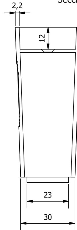
Sección C-C
